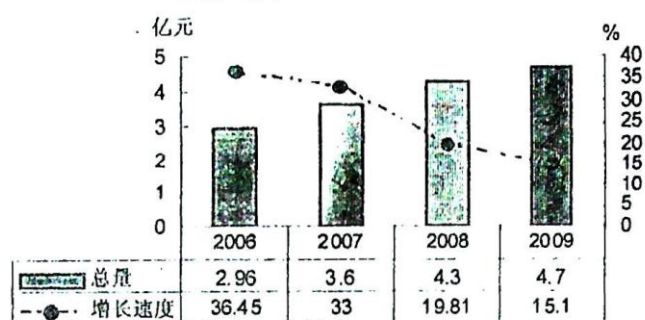
2006-2009年规模以上工业增加值总量、增速图
